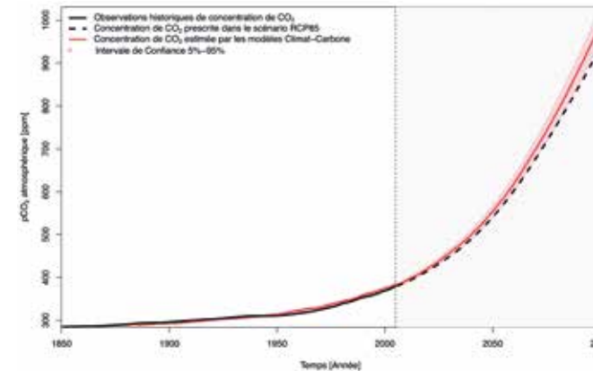
► Évolution du CO 2 atmosphérique observé de 1850 à 2006 puis projeté selon le scénario RCP8.5 jusqu'en 2100 et simulé par les modèles climat-carbone.
