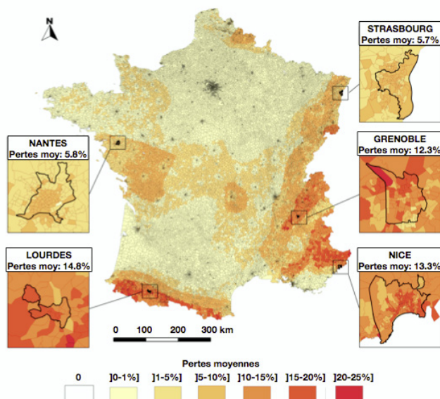
Dommage en pourcentage de la valeur du bien pour un aléa de période de retour 475 ans , obtenu par la méthode URBASIS - Riedel and Guéguen, Natural hazards, 2018
