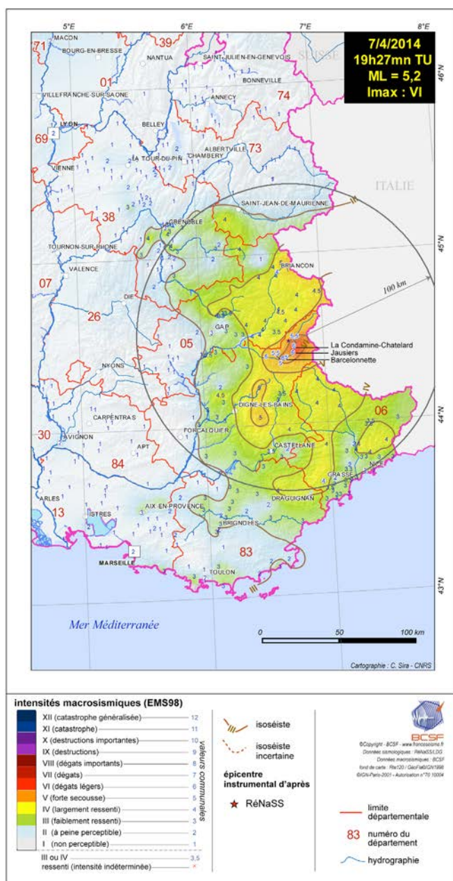
Carte d'iso-intensité établie par le Bureau Central Sismologique Français suite au séisme du 7 Avril 2014 (Ubaye). Intensité VI (Source BCSF)
